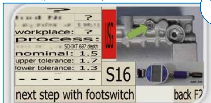
1 exemple d'une gamme de contrôle avec DIA-Gauge Esempio di "Sequenza guidata" con software DIA-Gauge
