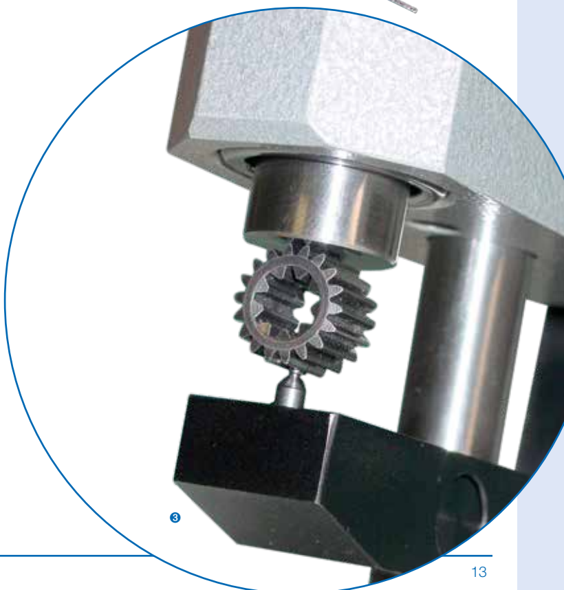
2 Mesures avec appareil AMG Misurazione di un D. E. 3 Contrôle de denture extérieure Controllo di dentatura esterna
