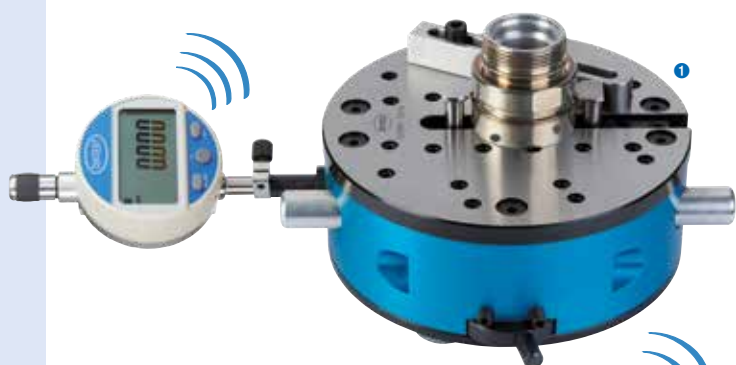
1 Table de mesure 2-points C2 2-punti tavolino di misura C2 2 Table de mesure 3-points C3-AL 3-punti tavolino di misura C3-AL 3 Table de mesure 2-points C2-JS 2-punti tavolino di misura C2-JS
