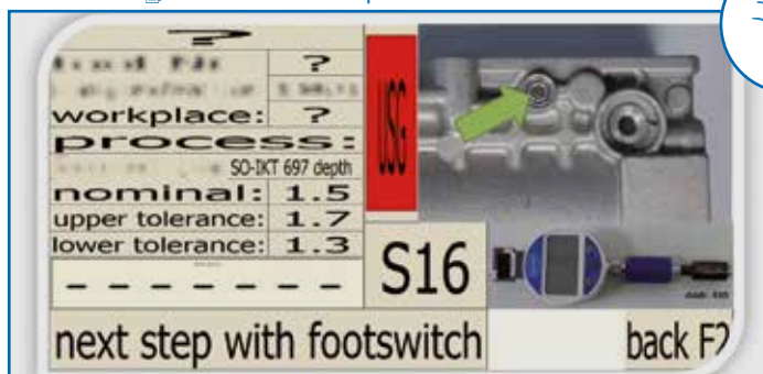
① exemple d'une gamme de contrôle avec DIA-Gauge Esemplio di "Sequenza guidata" con software DIA-Gauge
